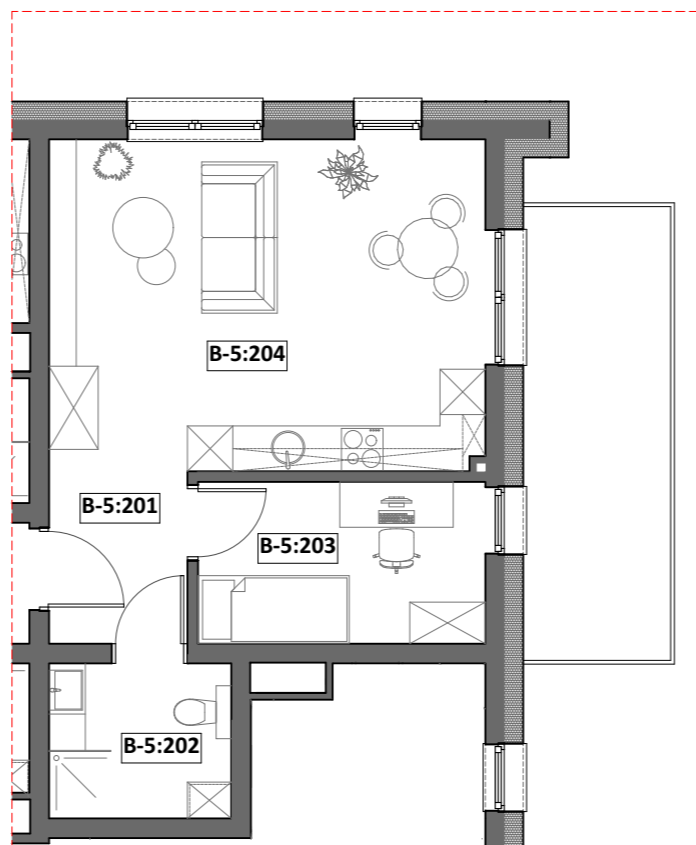
1 PIĘTRO - KLATKA B MIESZKANIA nr B-5
